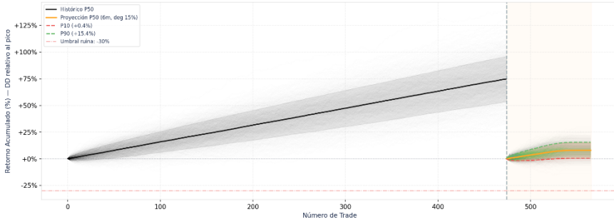
Histórico → Proyección (6m) | Degradación edge 15%
