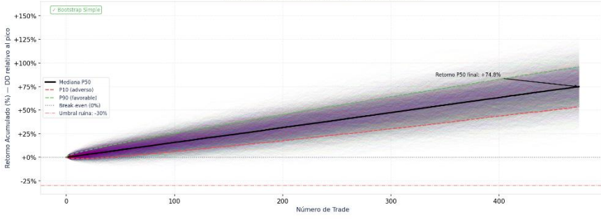
Distribución de Curvas de Retorno — Período Histórico
