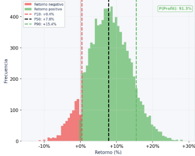
Distribución Retorno Final (6m)
