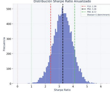
Distribución Sharpe Ratio Anualizado
