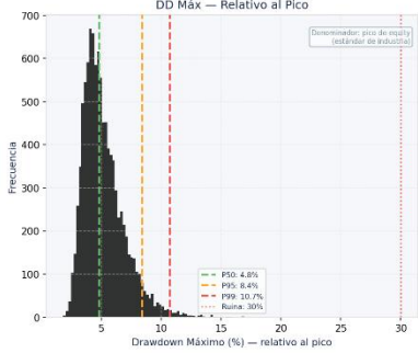
DD Máx — Relativo al Pico
